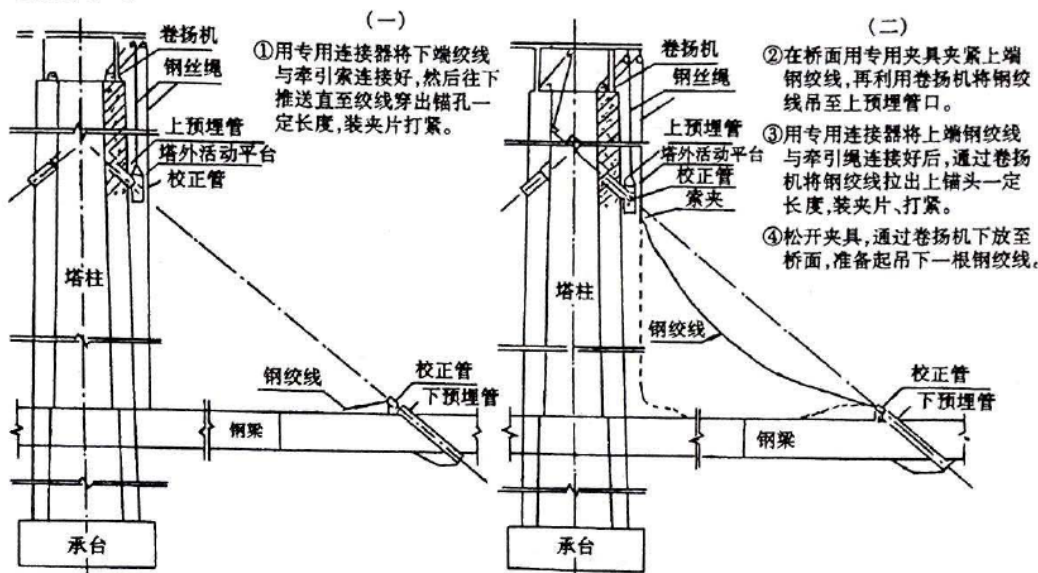
图3 岩石大桥单根挂索工艺示意图
