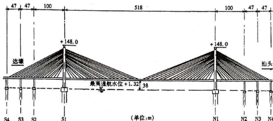
图2 宕石大桥主桥总体布置图
