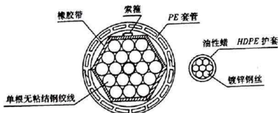
图 4 斜拉索 PE 套管及索断面图
