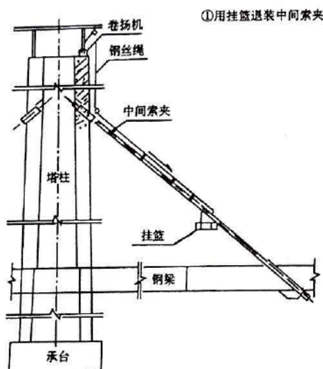
图 5 岩石大桥斜拉索索箍安装图
