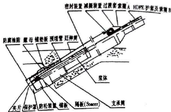
图1 锚具组件结构图
