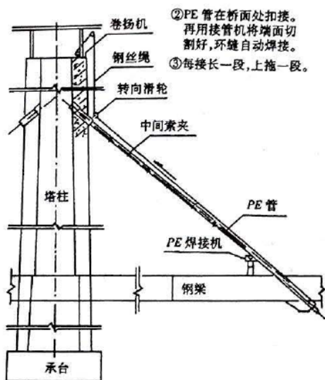
图 6 岩石大桥斜拉索 PE 套管安装图
